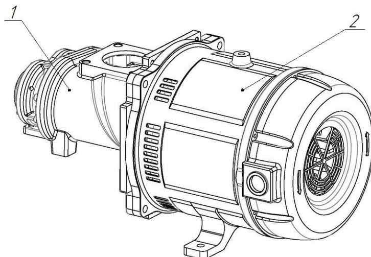
Рисунок 17 – Агрегат компрессорный
